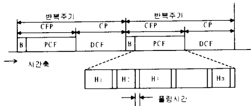
(그림 2) 무선 LAN의 시간축
