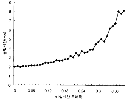
(그림 5) 비실시간 트래픽에 따르는 응답시간
