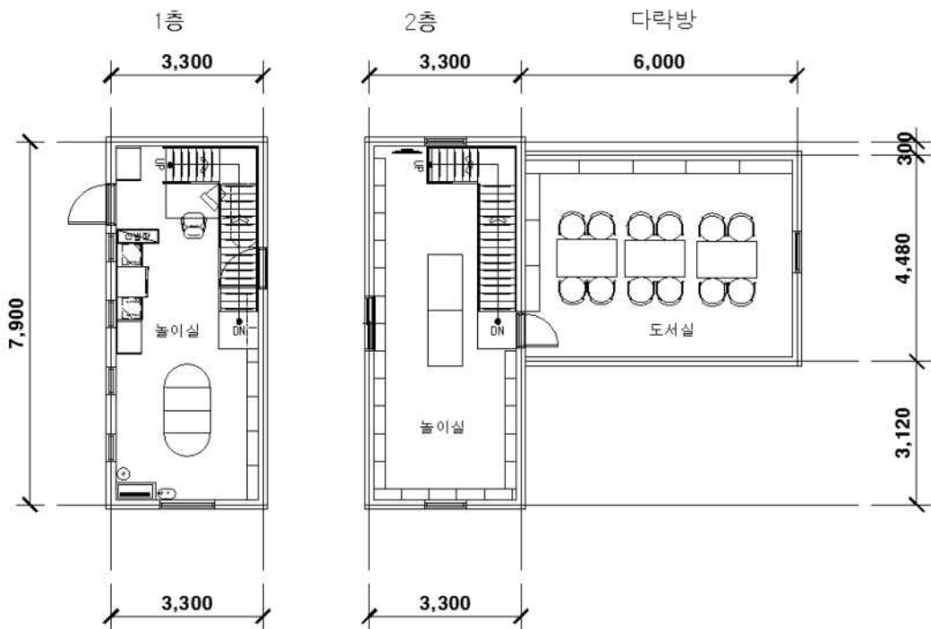
E호점 평면도 축척 : 1/100
