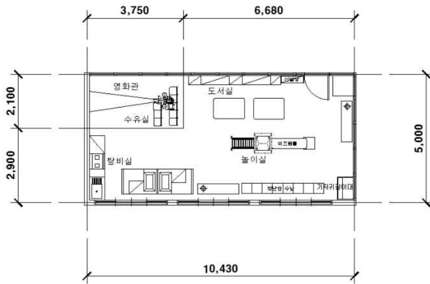
B호점 평면도 축척 : 1/100
