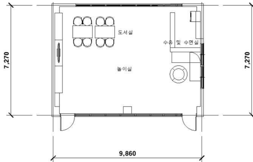
J호점 평면도 축척 : 1/100
